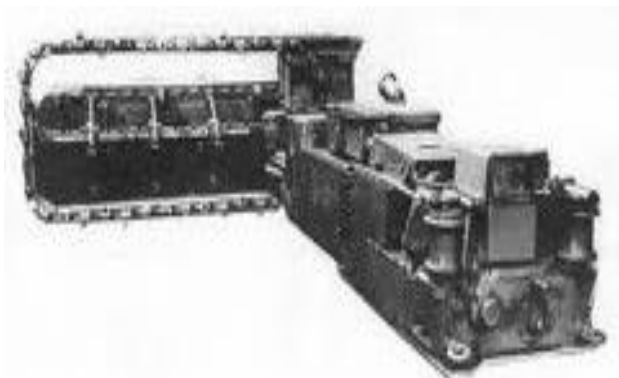
Очистной комбайн типа «Донбасс», сконструированный на основе изобретения А.Бахмутского
