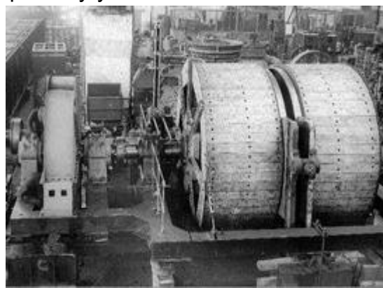
Сборка первой шахтной подъемной машины на НКМЗ, 1935 г.
